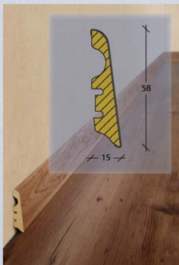
Ktex 1 15 x 58 x 2400 mm
