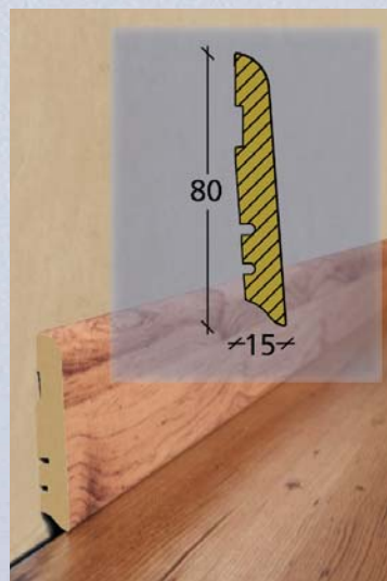
Ktex 6 15 x 80 x 2400 mm
