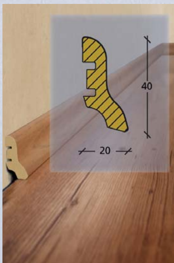
Ktex 4 20 x 40 x 2400 mm
