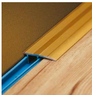
ЗАМЫКАЮЩИЙ ПРОФИЛЬ 7–13 мм, Длина: 2700 мм / 900 мм
