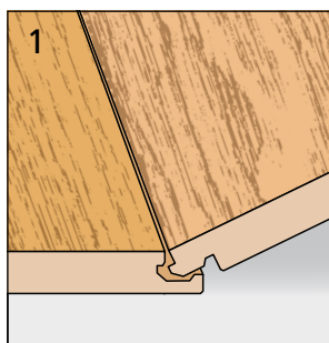
perfil longitudinal
