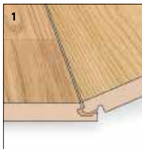
perfil longitudinal
